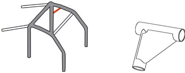
U-Förmiges Knotenblech
